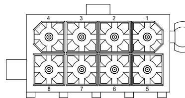
2X4PIN
