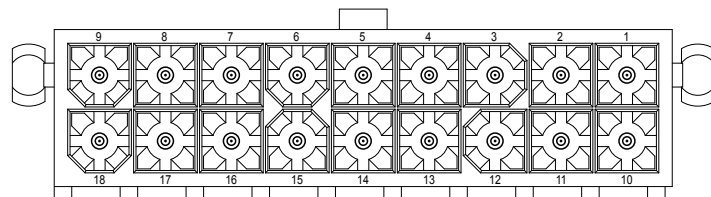
2X9PIN
