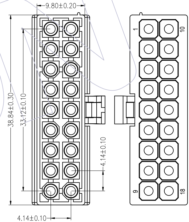
2X9PIN
